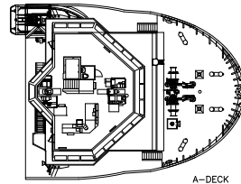
A-DECK
